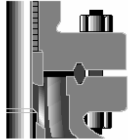
环连接面密封形式
